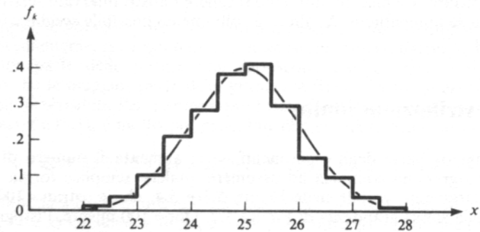
Figura 5.4. Istogramma per 1000 misure della stessa grandezza di Figura 5.3. La curva tratteggiata è la distribuzione limite.
