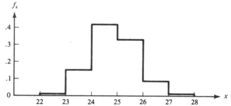
Figura 5.3. Istogramma per 100 misure della stessa grandezza di Figura 5.2.
